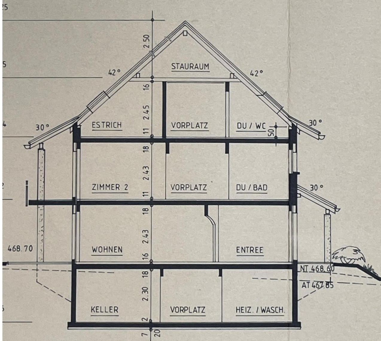
QUERSCHNITT HAUS 2 ST
